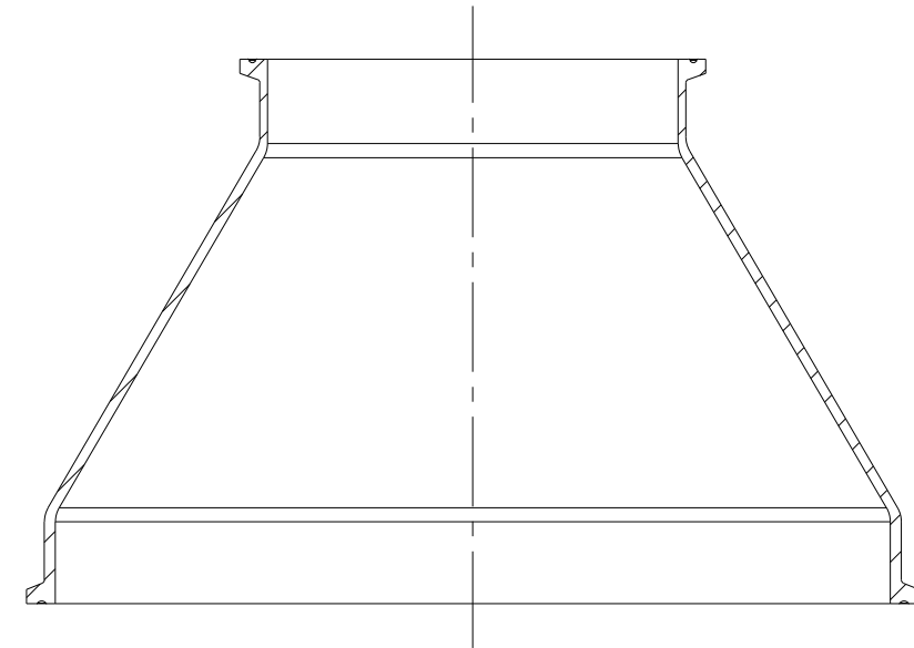
SECTION A-A SCALE 1:3
